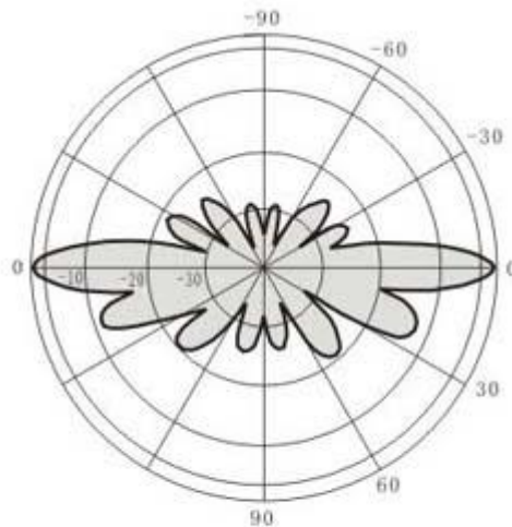
垂直面方向图 Vertical Plane
